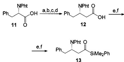
Scheme 5. a) ref. [30] , 90%; b) CH 2 N 2 , Et 2 O/THF, r.t., 1 h, 94%; c) Ag 2 O, MeOH, 50°C, 40 min, 87%; d) HCl, H 2 O, acetone, reflux, 150 min, 81%; e) SOCl 2 , 55°C, 4 h, 93%; f) (PhMe 2 Si) 2 CuCN(Li) 2 , –78°C, 1 h, 55%
